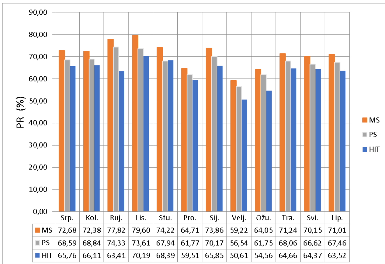
Slika 5.1. PR fotonaponskih modula u postocima
