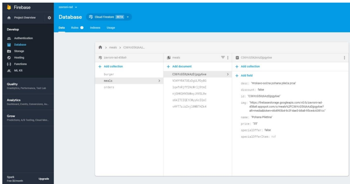
Slika 3.9. Firebase sučelje.
