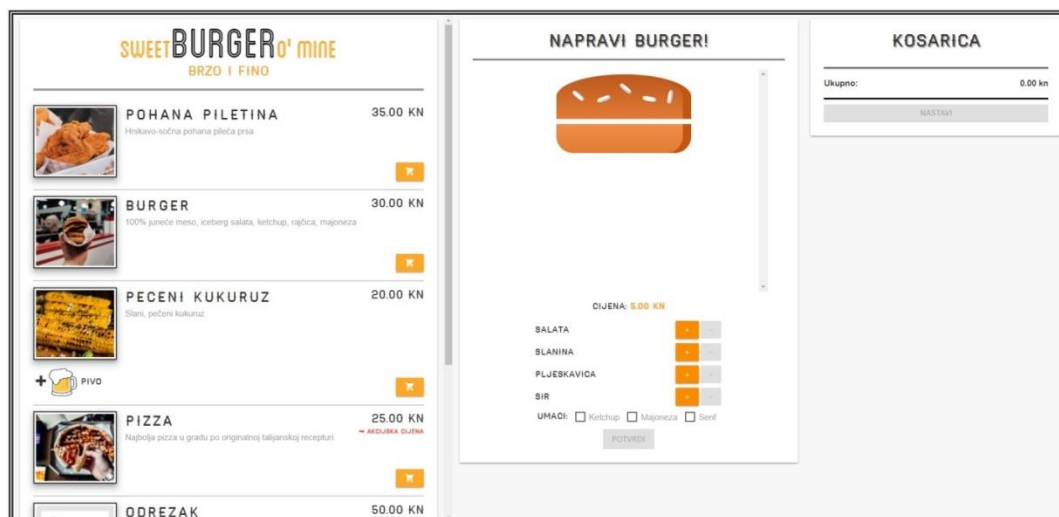
Slika 3.6. Korisničko sučelje.
