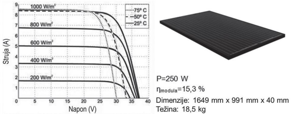
Slika 5.1 strujno naponska karakteristika fotonaponskog modula[9]
