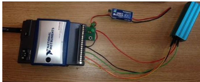
Slika 7.6. ADXL330 akcelerometar spojen sa mjernim čvorom NI WSN – 3202
