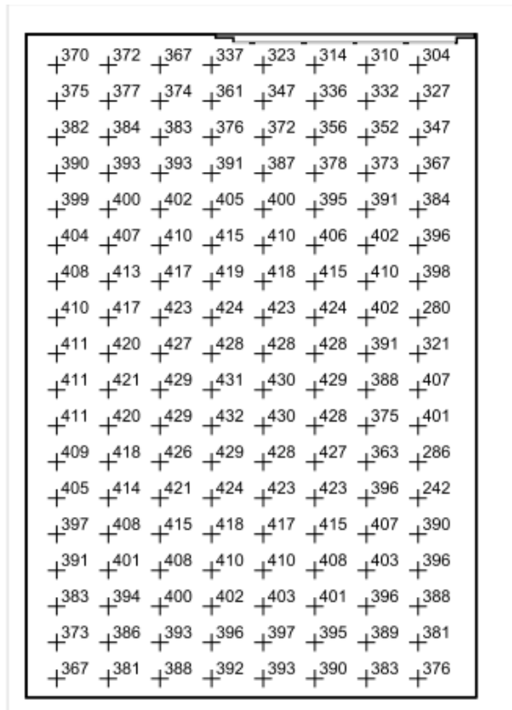
Scale: 1 : 25
