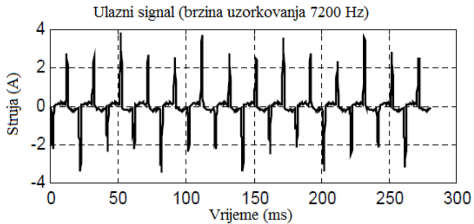
Slika 6.23. Međuharmonici (Švedska) [8]
