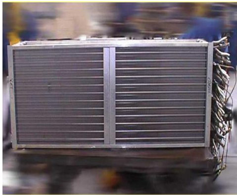
Slika 4.7. Prikazuje uspravnu izvedbu rekuperacije zraka pomoću toplinskih cijevi i izgled u praksi. Veći broj cijevi omogućuje i veću učinkovitost sustava što rezultira većim povratom topline, [12].
