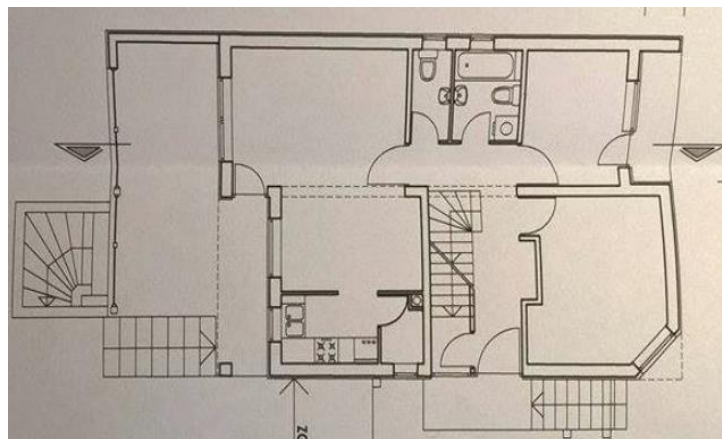
Slika 6.4. Tlocrt prizemlja obiteljske kuće.
