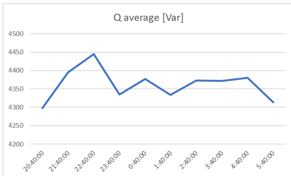
Slika 4.20. Grafikon mjerenja jalove snage
