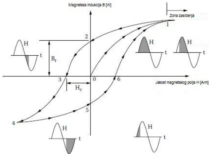
Slika 2.5. Krivulja petlje histereze;[5]
