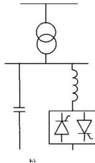
Slika 3.2. Tiristorski kontrolirana zavojnica sa filtrom;[6]
