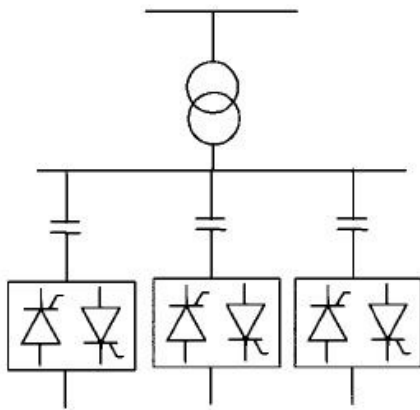
Slika 3.3. Tiristorski paljeni kondenzato;[6]
