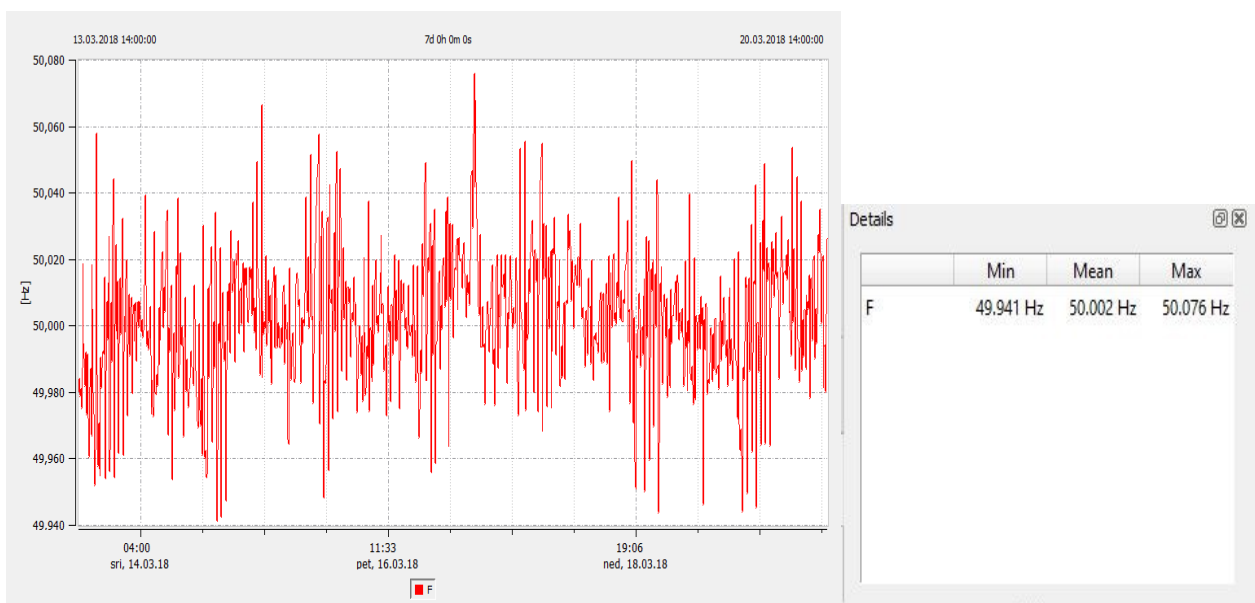
Slika 4.4. Analiza frekvencije
