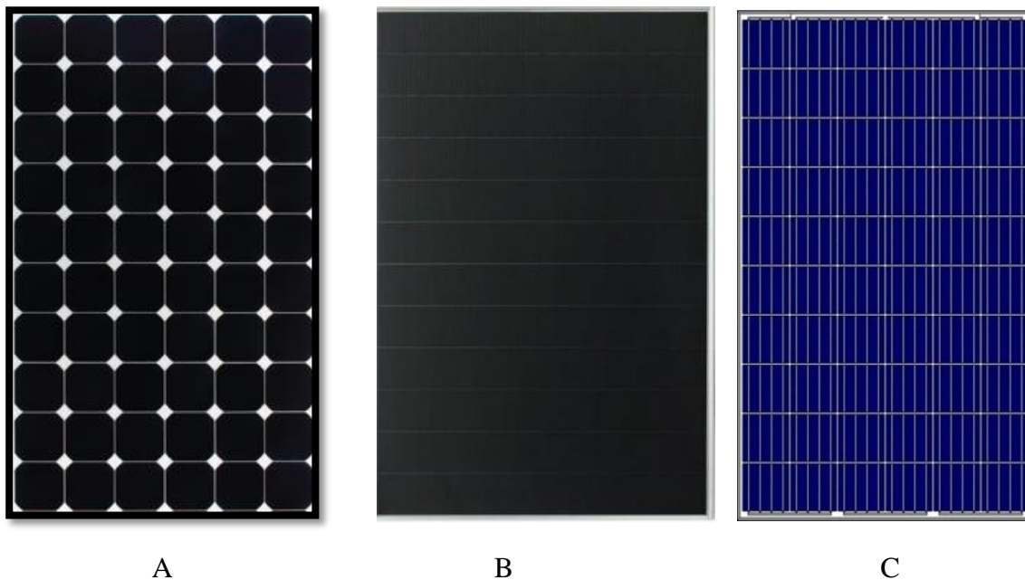
Slika 4.6. izgled fotonaponskih modula ovisno o tehnologiji izvedbe: A) monokristalni silicijski, B) tankoslojni, C) polikristalni silicijski fotonaponski modul
