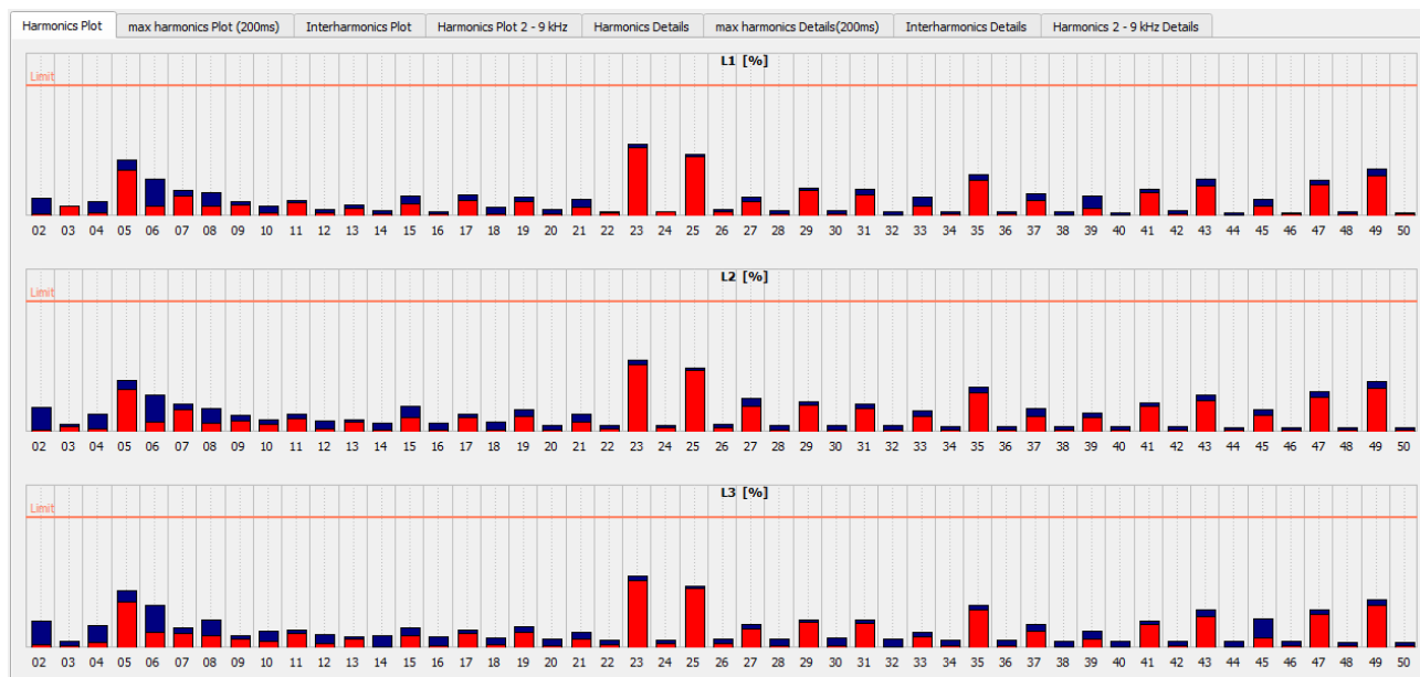
Slika 4.5. Naponi viših harmonika
