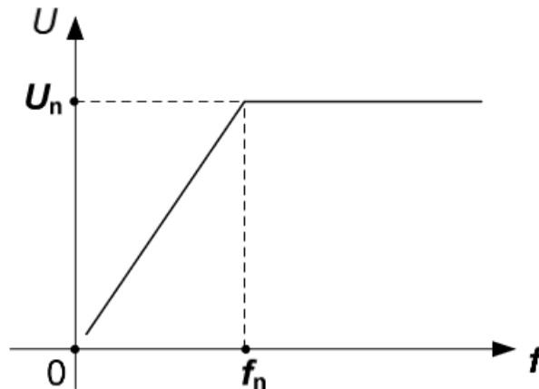
Slika 2.18. Grafički prikaz promjene napona i frekvencije kod skalarne regulacije [7].
