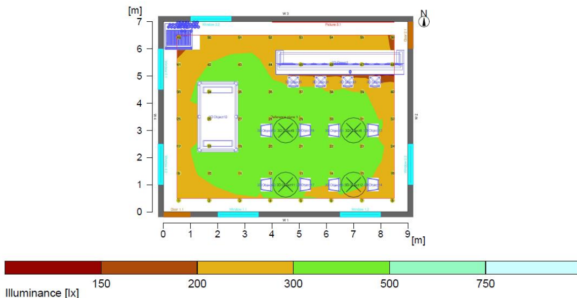
Slika 5.3. Svjetlotehnički proračun[P.5.1.]
