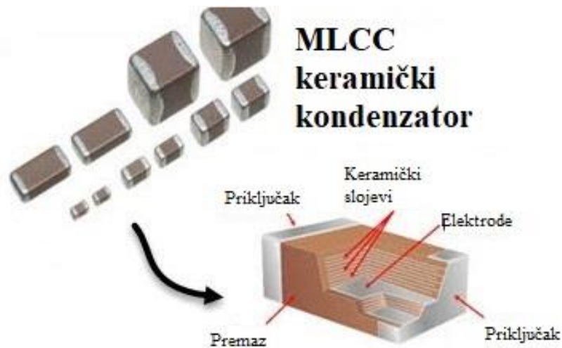
SI.4.4. Višeslojni keramički kondenzator
