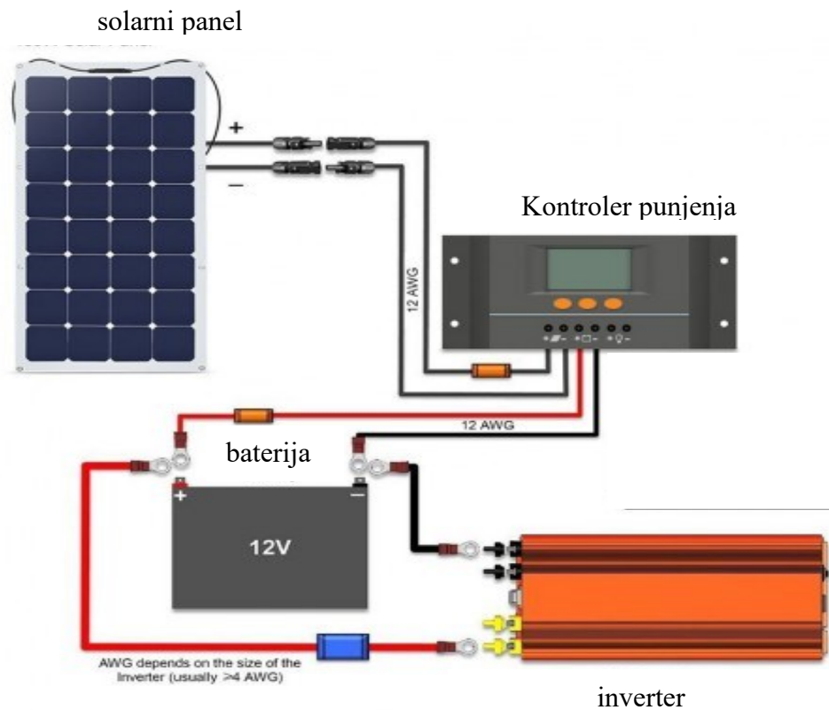
Slika 4.6. Način rada elemenata fotonaponskih sustava [11]
