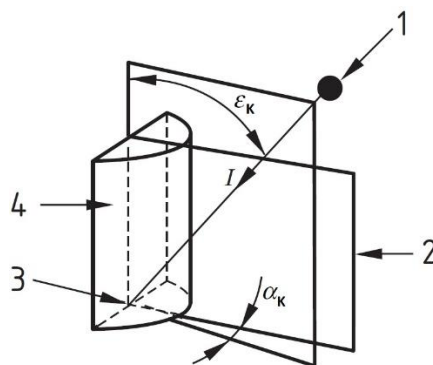
Slika 3.5. Kutovi za proračun polu-cilindričnog osvjtljenja [13].
