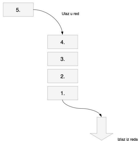
Slika 2.4. Prikaz algoritma FIFO [5]
