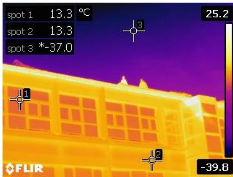
Sl.3.1. Primjer termograma zgrade
