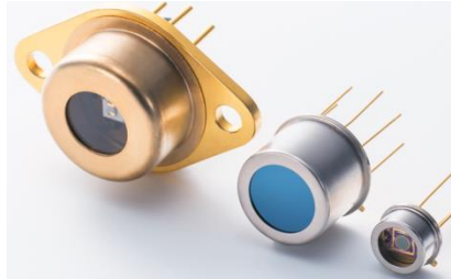
SI.2.3. Različiti infracrveni detektori (s lijeve strane: InSb, InAsSb, InGaAs ) [5]
