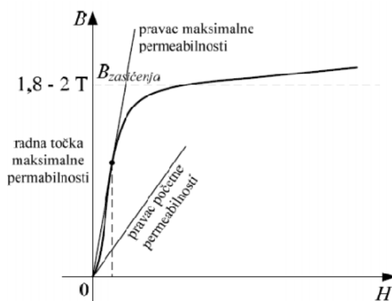
Slika 4.2. Krivulja magnetiziranja [4]
