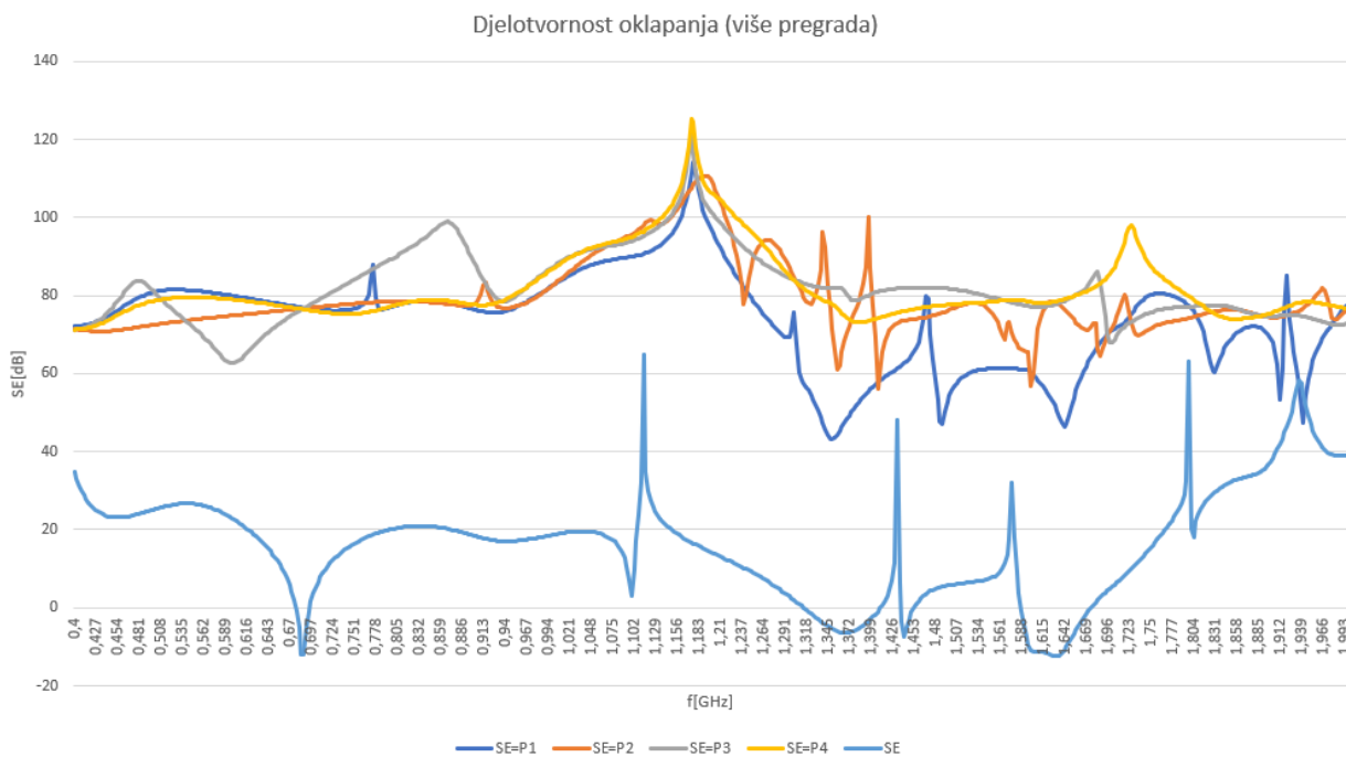
Slika 3.12. Rezultati simulacije sa većim brojem identičnih pregrada.
