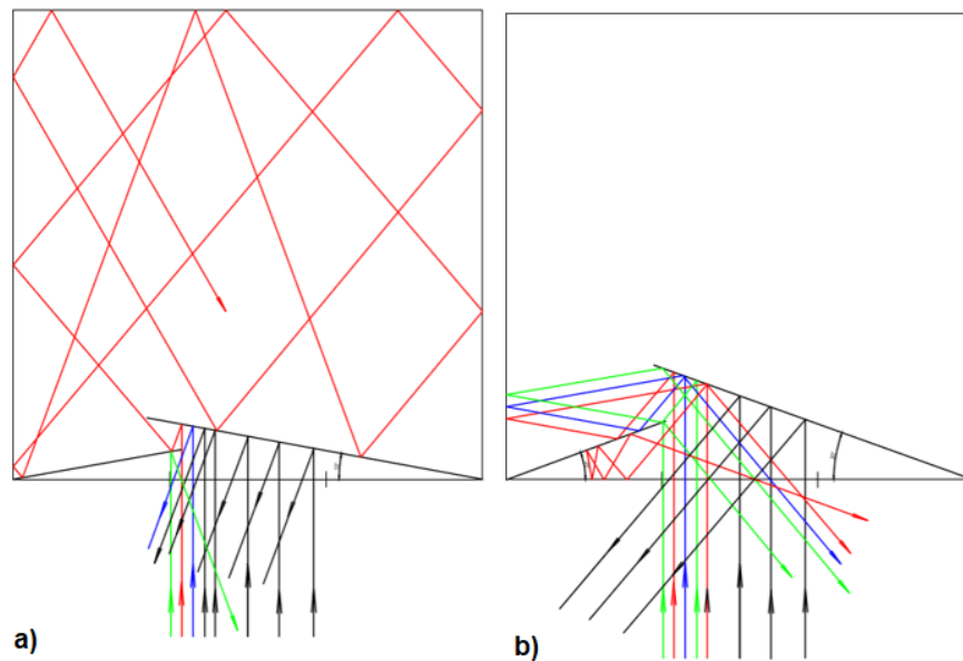
Slika 2.9. a) oklop sa velikom i malom pregradom 10^\circ , b) oklop sa velikom i malom pregradom 20^\circ
