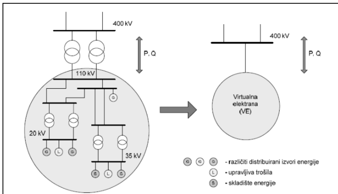
Slika 2.14. Virtualna elektrana [20]
