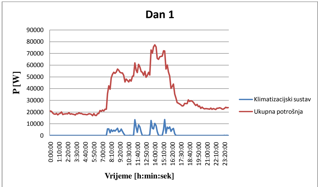
Slika 4.4. Ukupna potrošnja električne energije zgrade i klimatizacijskog sustava prvog dana
