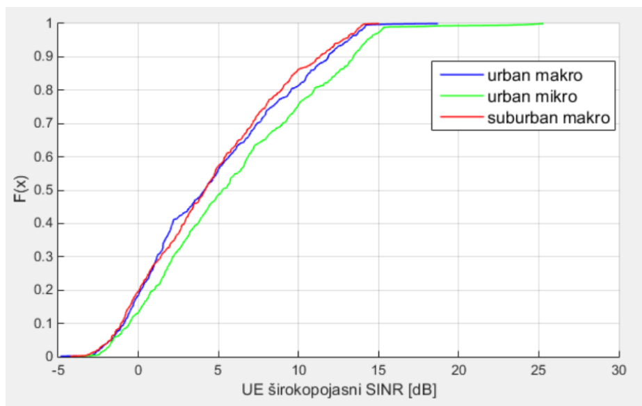
Sl.4.13. Prosječni UE širokopojasni SINR
