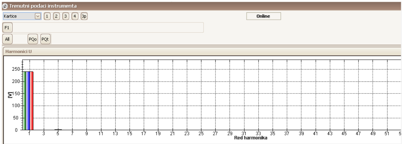
Slika 3.1.11. Harmonici napona za transformator u normalnom stanju rada
