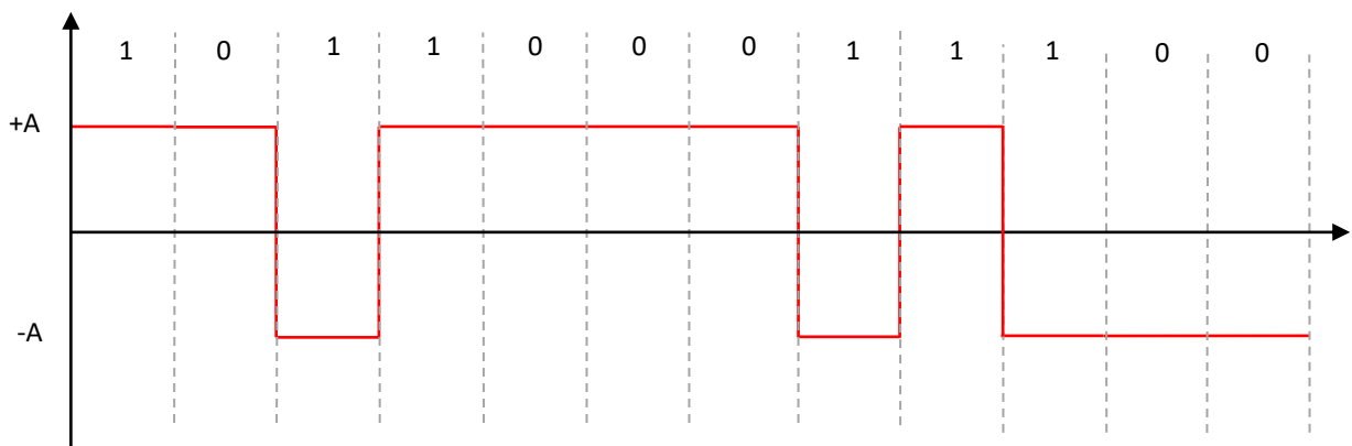
Slika 2.10. Oblik NRZ-M
