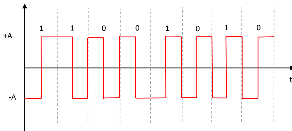
Slika 2.14. Primjer DIFERENCIJALNOG MANCHESTER koda
