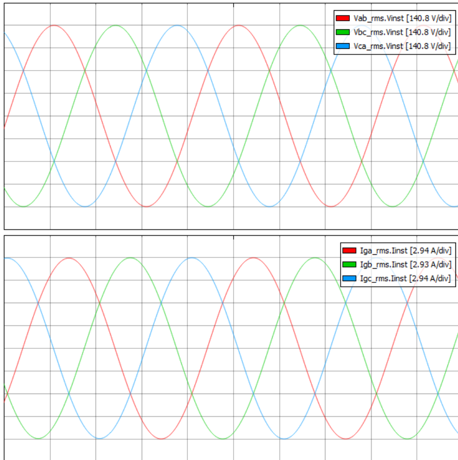
Slika 5.15. Slučaj 1b: Prikaz osciloscopa pri velikom opterećenju
