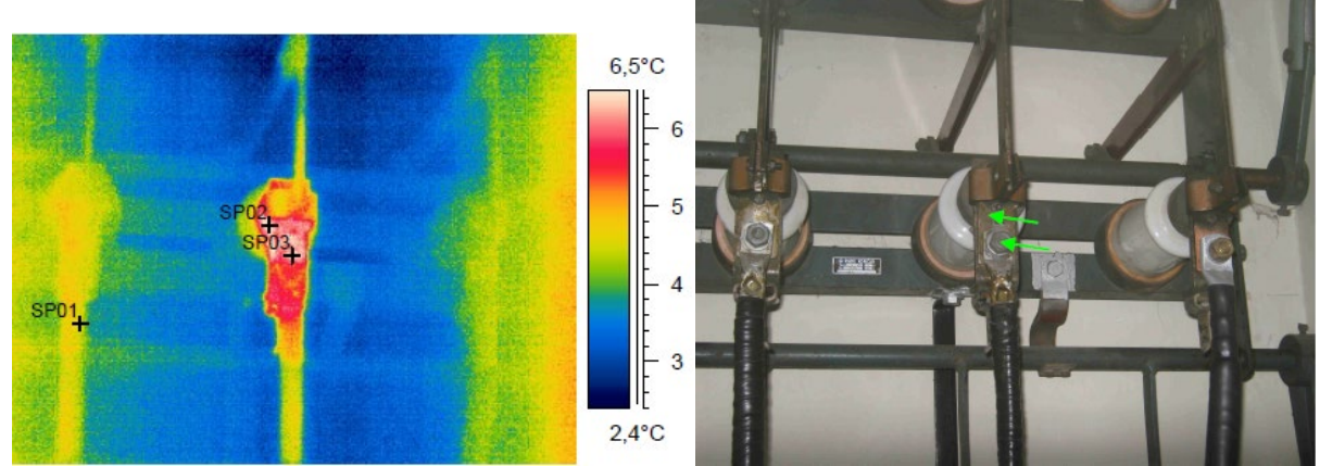
Slika 7.53. TS 35/10 kV - ZAPAD
