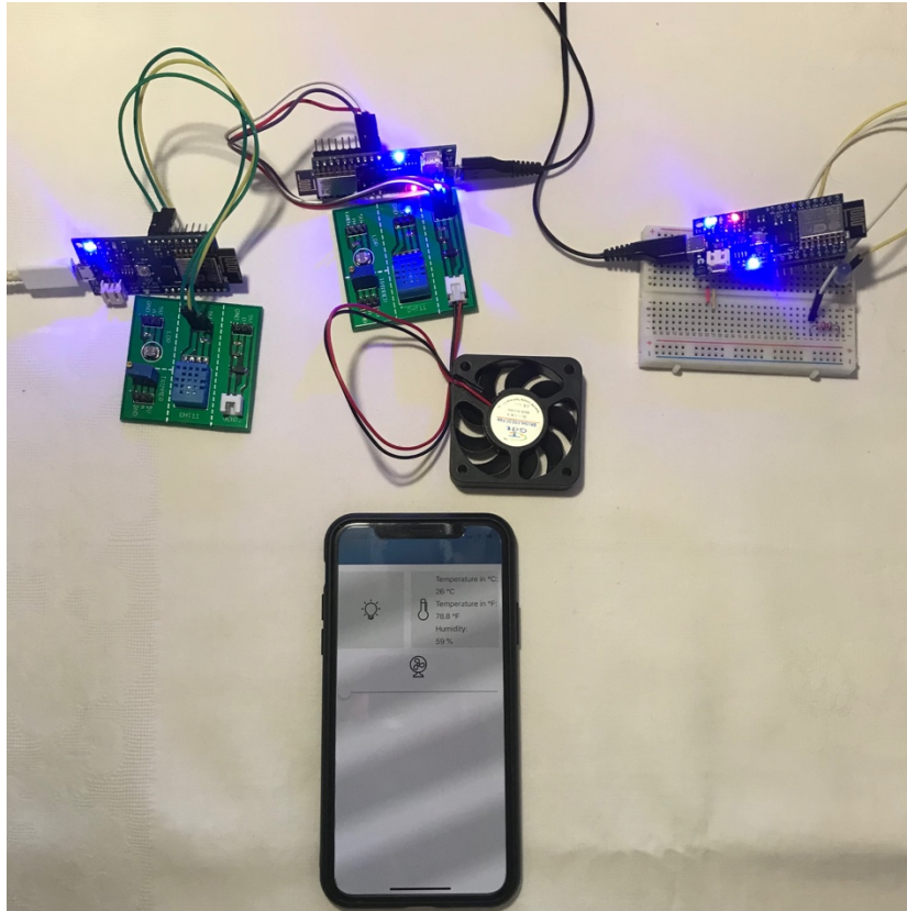
Slika 3.4. Fotografija testiranja aplikacije i Croduino uređaja.
