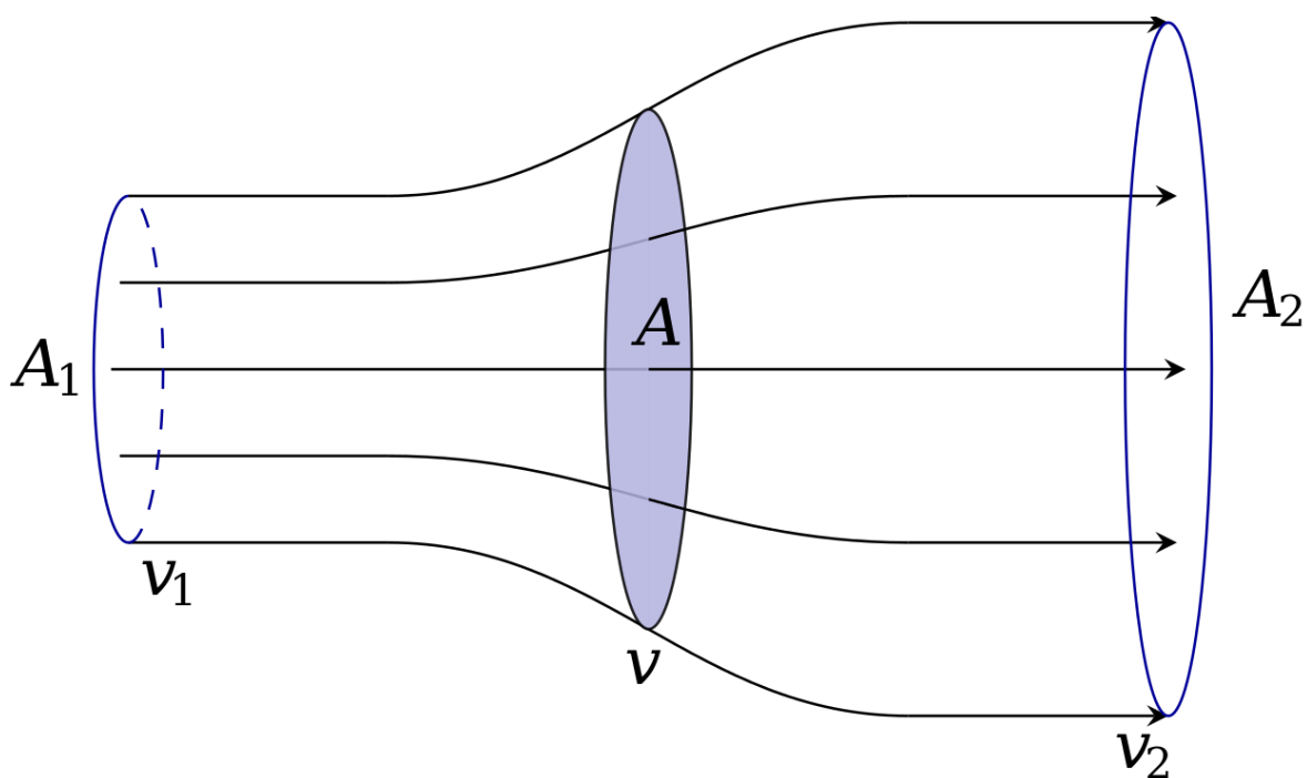
Slika 1.21. Betzov difuzor [11]
