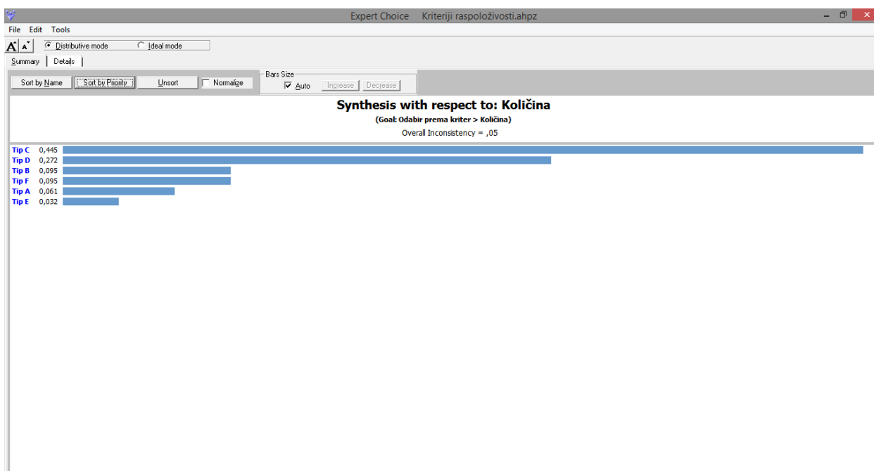
Slika 5.12. Prioriteti najoptimalnijih tipova elektroagregata prema količini
