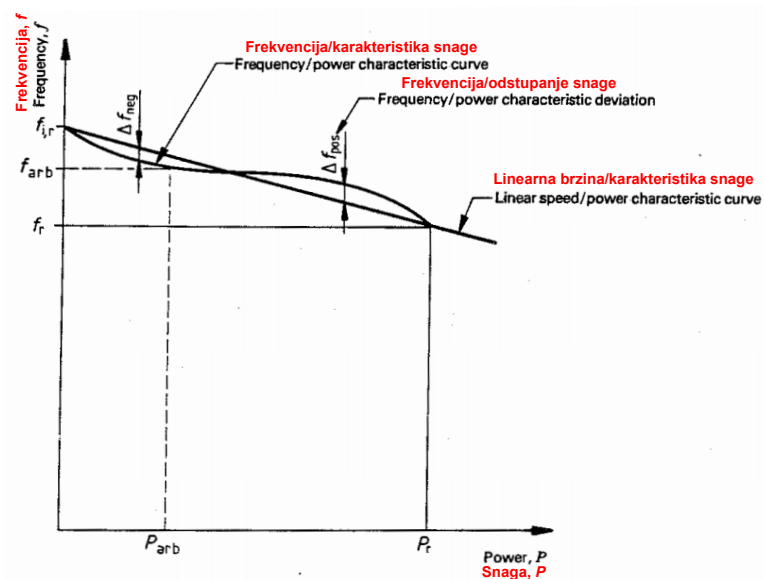
Slika 3.2. Devijacija frekvencije od linearne karakteristike pri promjeni opterećenja od praznog hoda do nazivne snage tereta [15]
