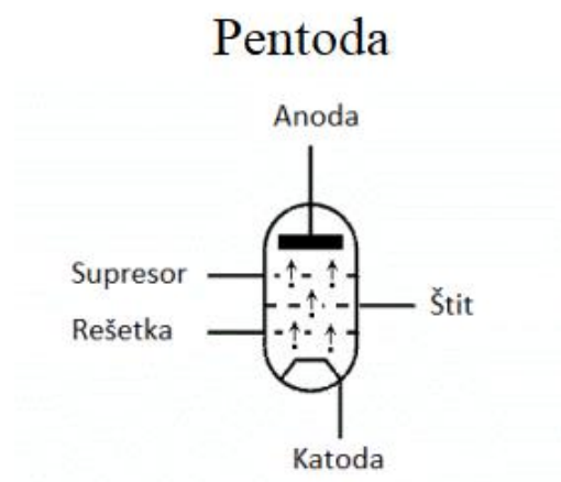
Slika 3.3. Pentoda
