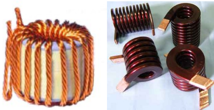
Slika 4.5. Namotaji s isprepletenim žicama bakra (lijevo) i ravnim žicama bakra (desno) [24]
