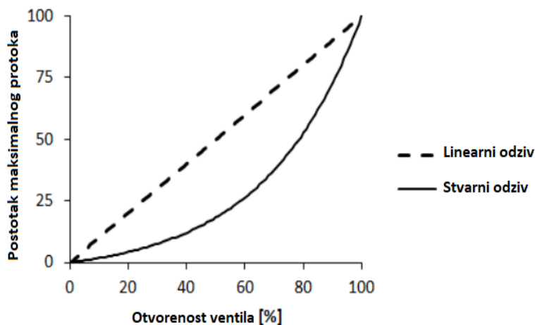
Slika 2.4. Ovisnost otvorenosti ventila o postotku protoka
