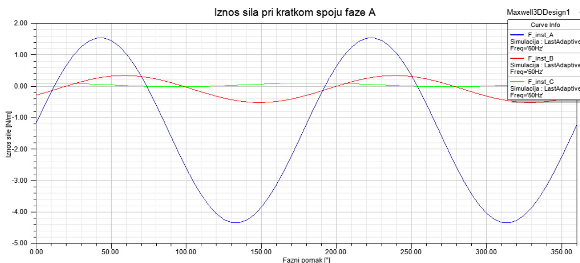
Slika 5.13. Iznos sila u sabirničkom sustavu pri kratkom spoju u fazi A u 3D modelu
