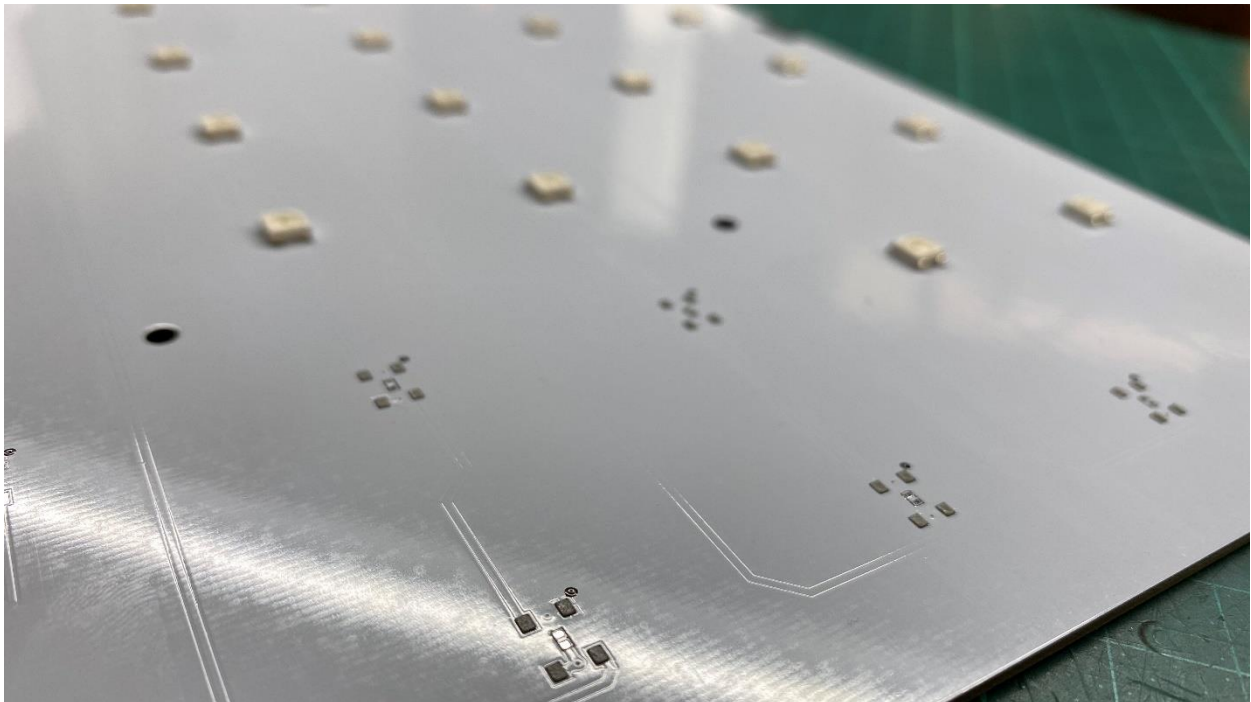
Slika 3.22: Završena tiskana pločica sa lemnom pastom
