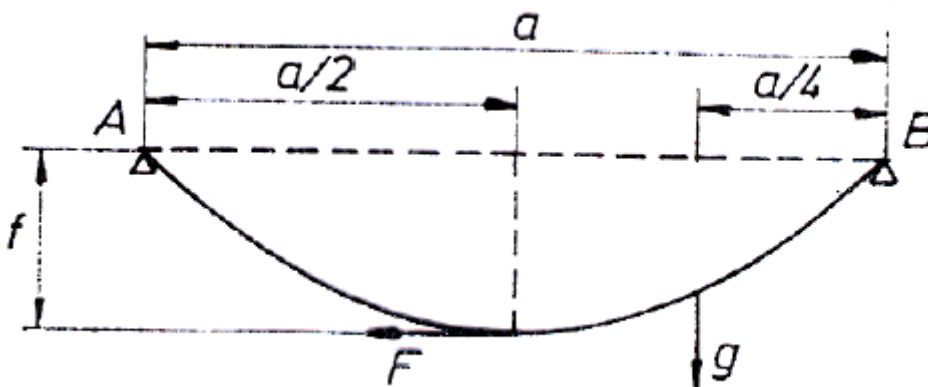
Slika 4.4. Ispitivanje ravnoteže zategnutog užeta pri ovjesištima nejednakih visina [4]
