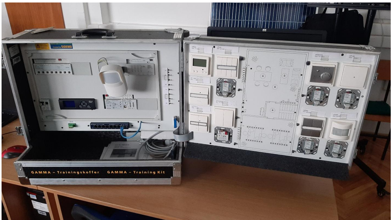
Slika 4.1. SIEMENS GAMMA sustav za vježbu-tvornička konfiguracija [Autorska fotografija]
