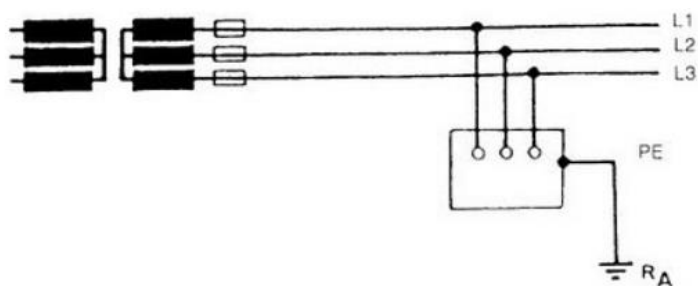
Slika 2.5: IT sustav [3]
