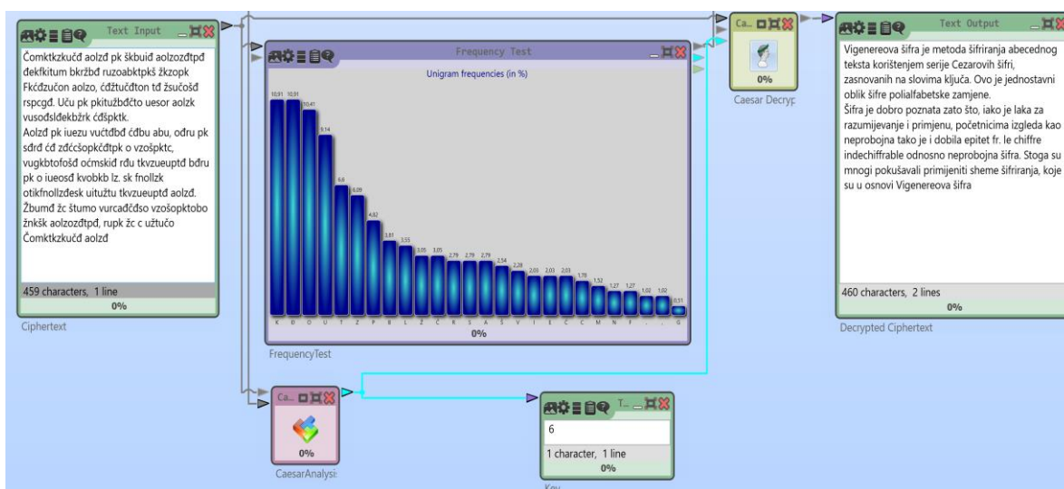
Slika 5.9 Primjer 3: Kriptoanaliza Cezarove šifre korištenjem frekvencije slova
