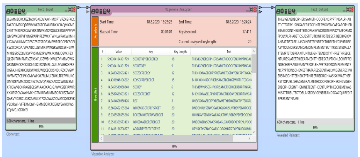
Slika 5.18 Primjer 1: Vigenerova analiza
