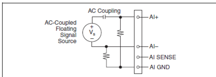
Slika 2.7.3. Diferencijalni spoj za izmjenični izvor s dva otpornika
