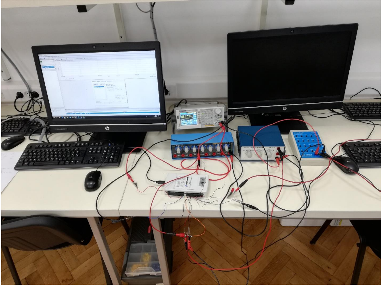
Slika 3.3.4. Slika spojenog serijskog RLC kruga s AD karticom
