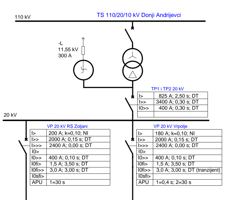
Slika 4.3. Podešenje relejne zaštite u TS 110/20/10 kV Donji Andrijevci [3]
