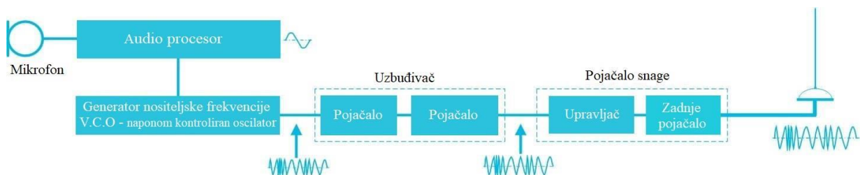
Slika 8. Princip rada FM predajnika
