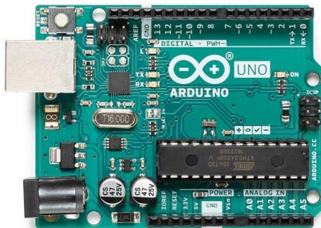
Sl. 3.1. Arduino Uno platforma [6]
