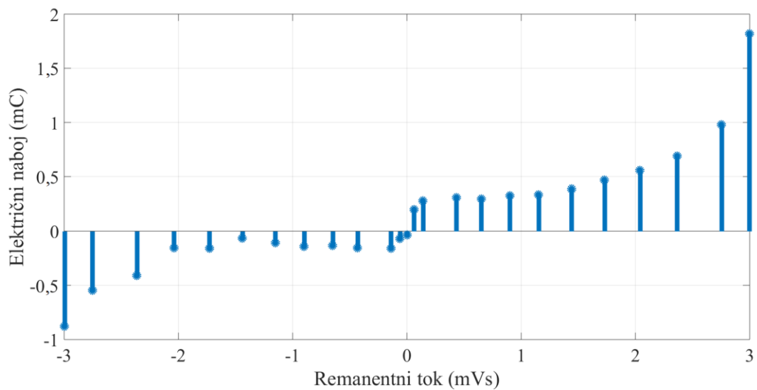
Slika 4.13. Vrijednosti električnog naboja ( Q ) za parametre E = 1 V, T = 20 ms i t_1 = 2T .
