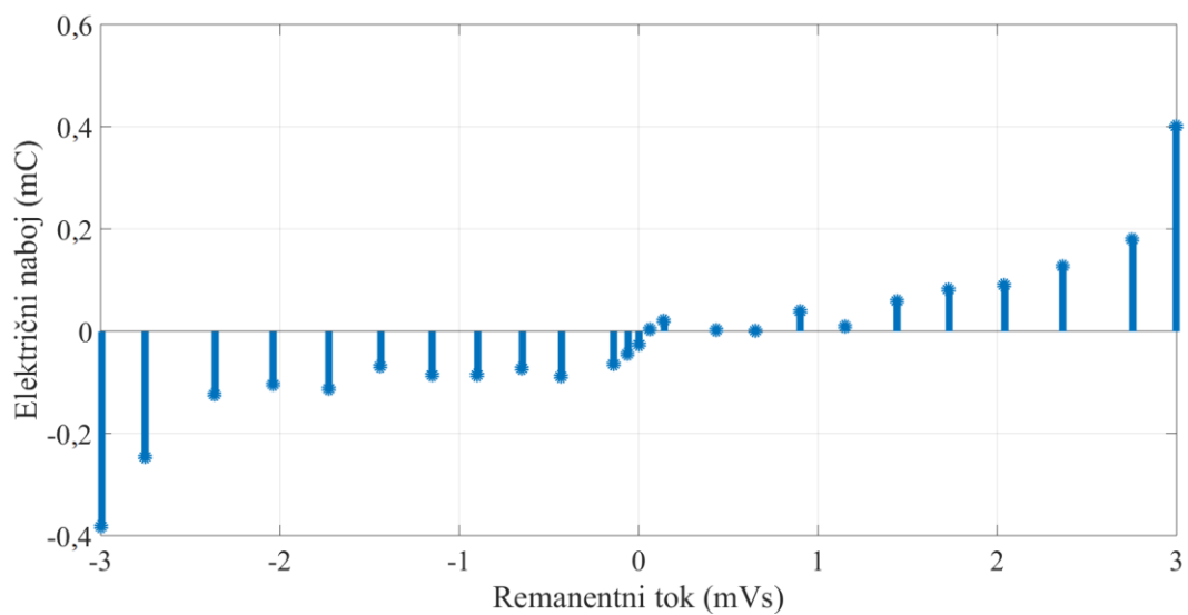
Slika 4.14. Vrijednosti električnog naboja ( Q ) za parametre E = 4 V, T = 5 ms i t_1 = 2T .
