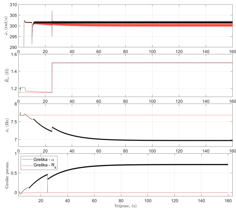
Slika 4.21: Adaptacija parametara - dugotrajno opterećenje, idealne struje, promjena R_s
