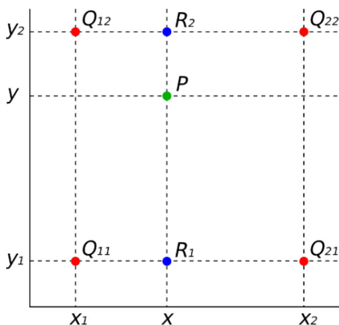
Slika 2.4. Bilinearna interpolacija
