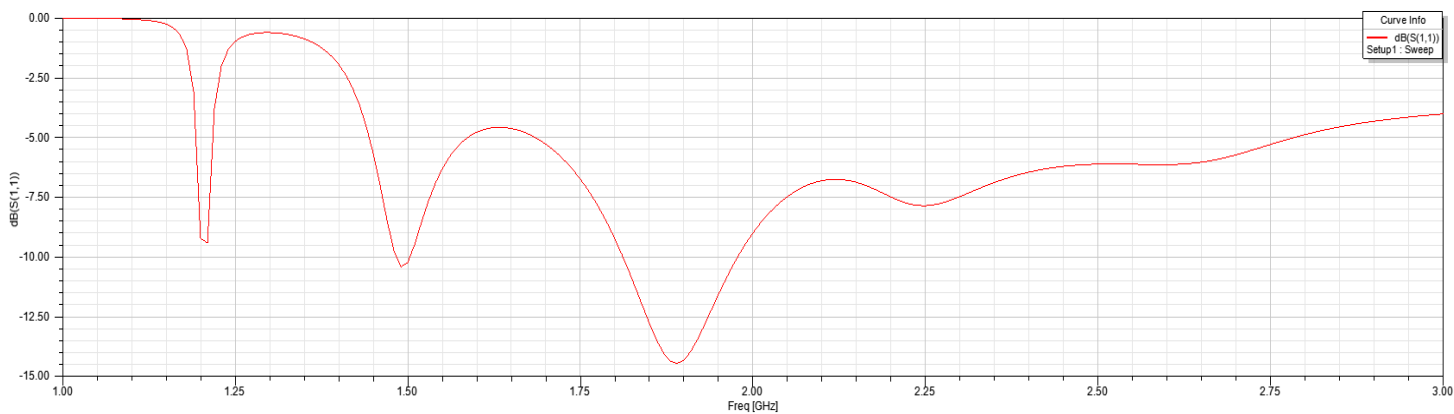
Sl. 5.2. S_{11} za D=6\text{cm} , N=4
