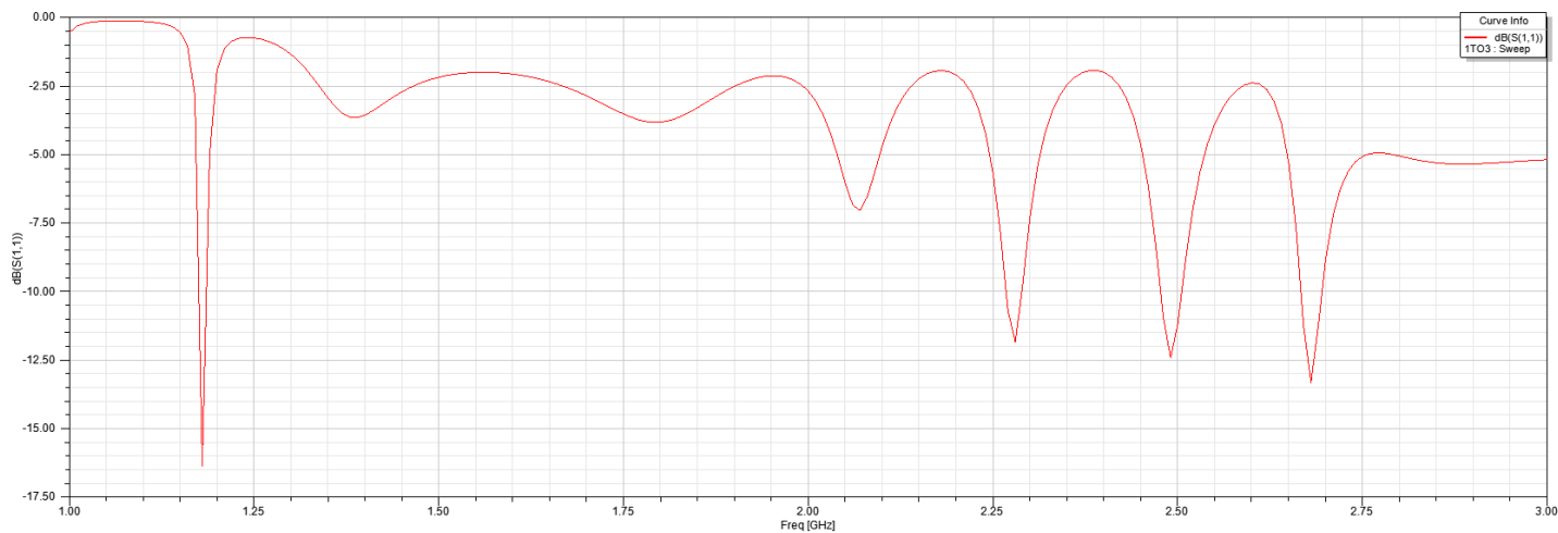
Sl. 7.2. S_{11} za helikoidalnu antenu ( D=6 cm, N=4 )
