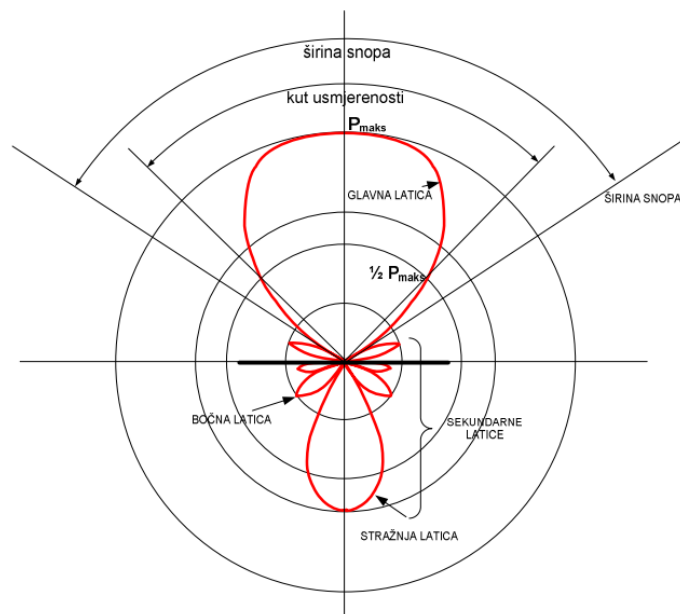
Sl. 3.4. Karakteristične veličine dijagrama zračenja
