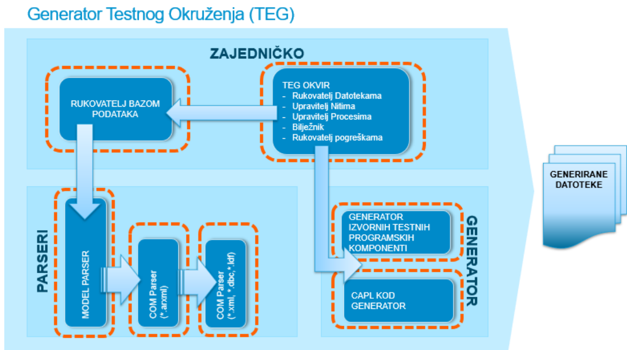
Slika 2.1: Blok dijagram konceptualne sheme TEG-a [2]
