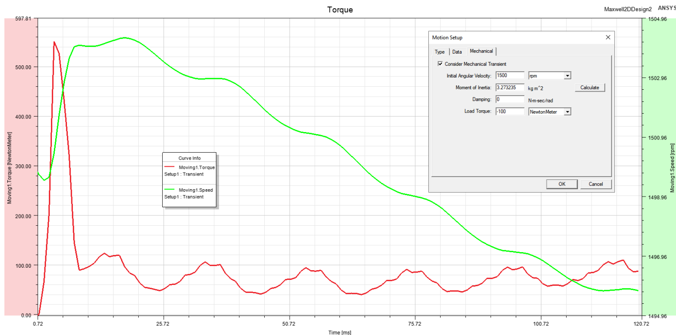
Slika 9.41. Simulacija zaleta motora s teretom od -100 Nm.
