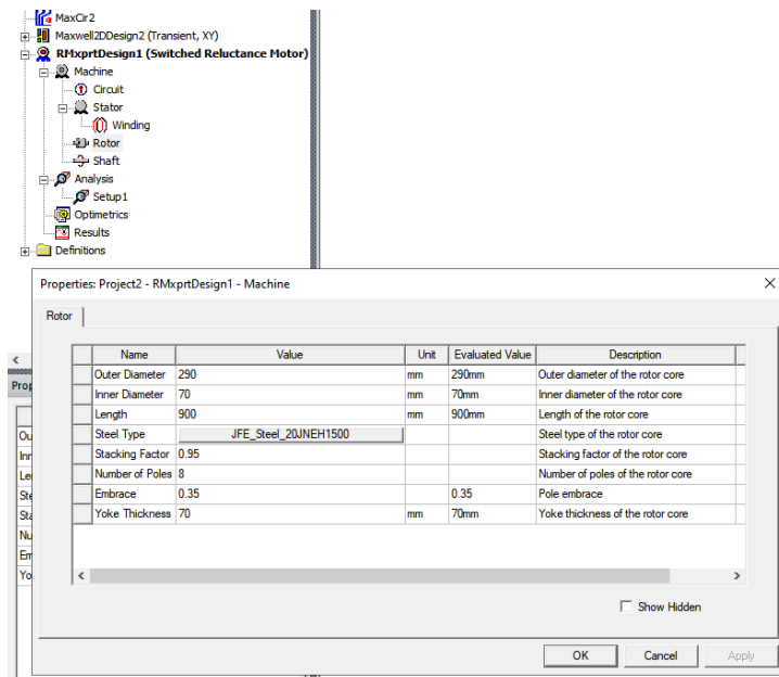
Slika 9.6. Određivanje parametara rotora motora.
