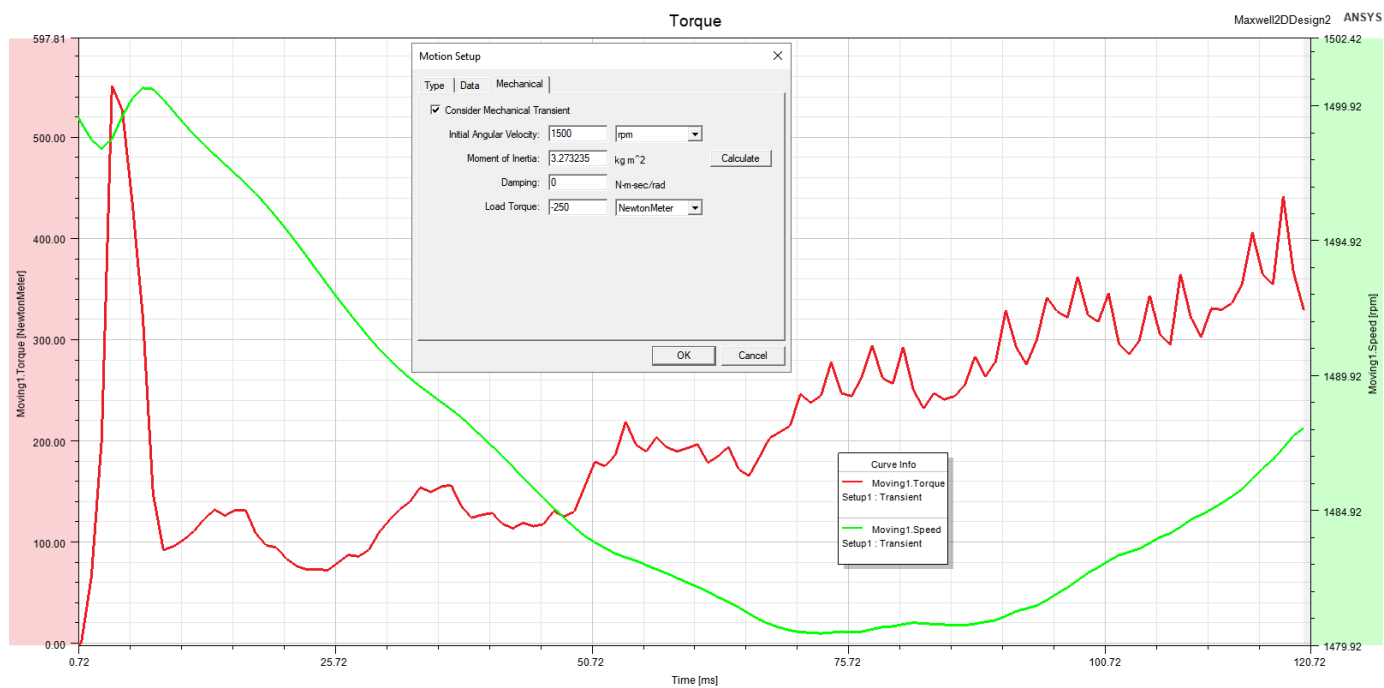
Slika 9.42. Simulacija zaleta motora s teretom od -250 Nm.
