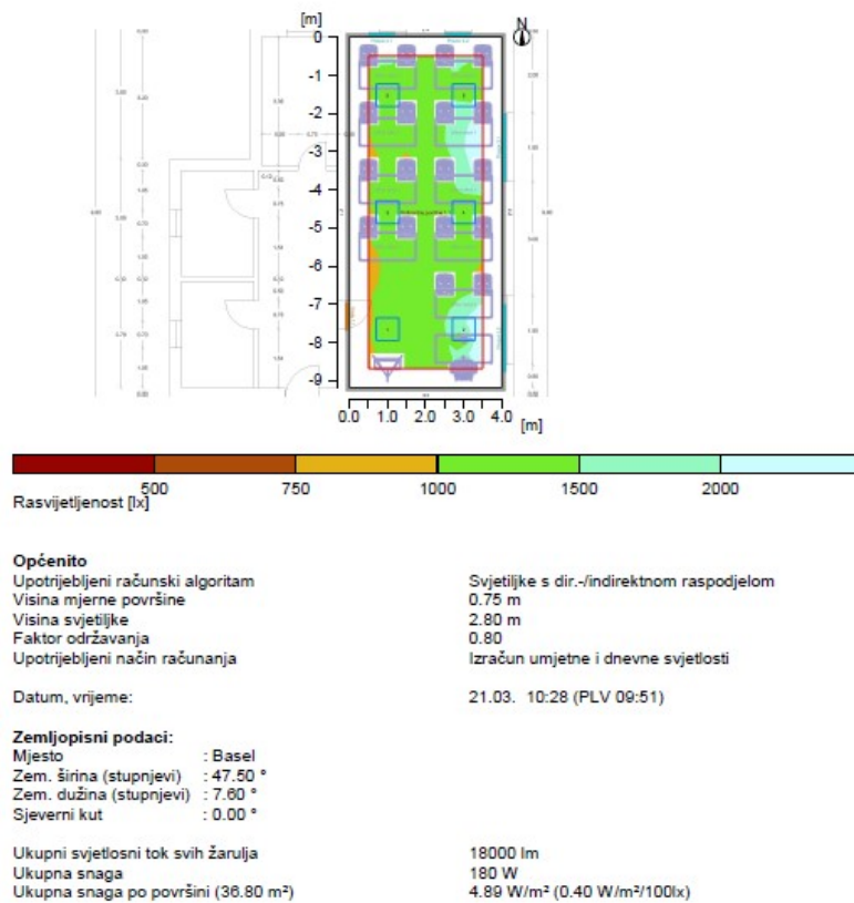
SI.6.15 Prikaz rasvjetljenosti predavaonice dnevnim i umjetnom rasvjetom
