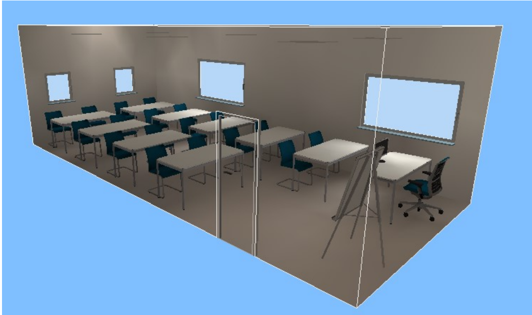
SI.6.10 3D prikaz rasvjetljenosti prostorije dnevnim svjetlom.
