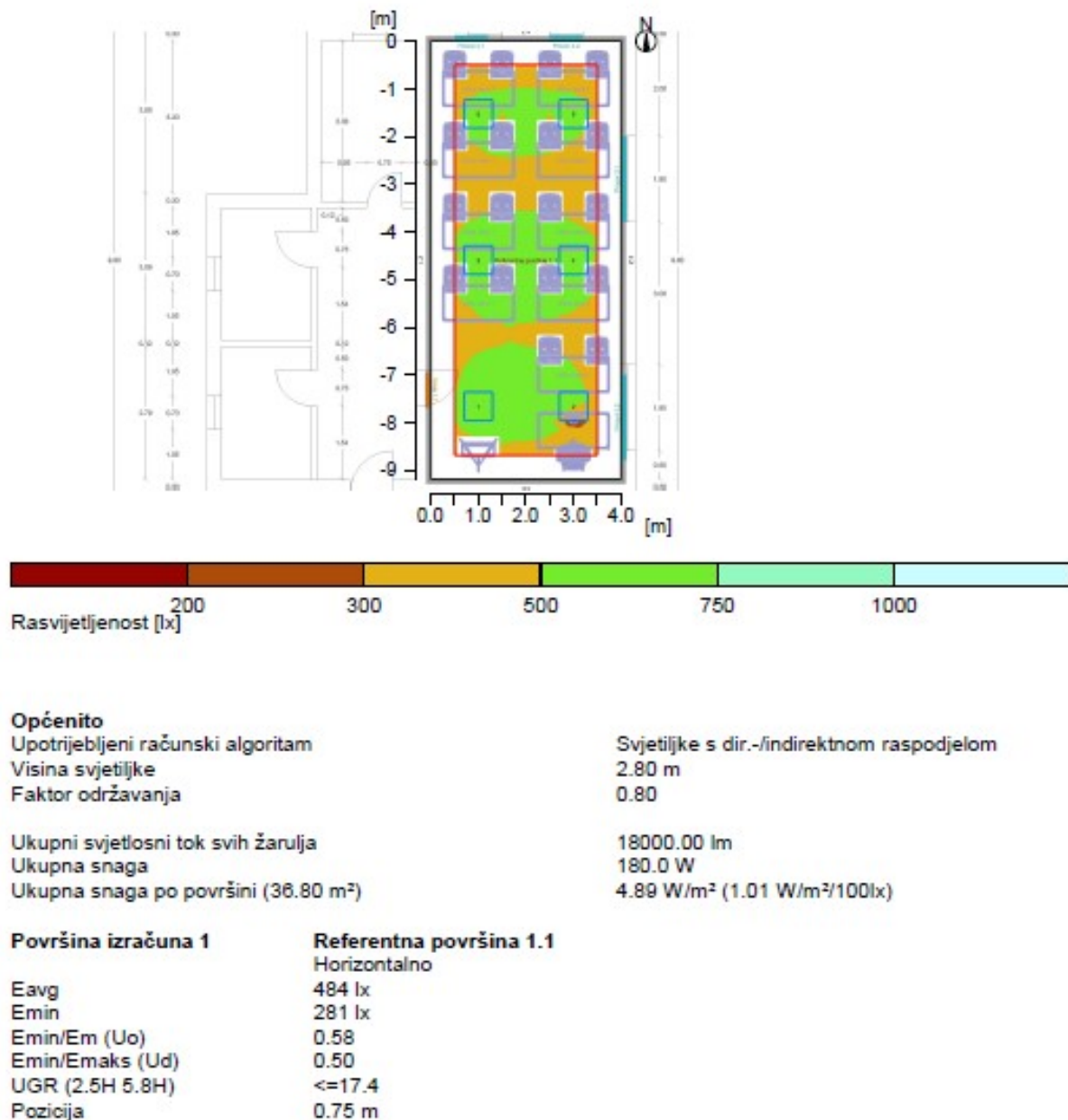
Sl.6.4. Prikaz rasvijetljenosti umjetne rasvjete za predavaonicu
