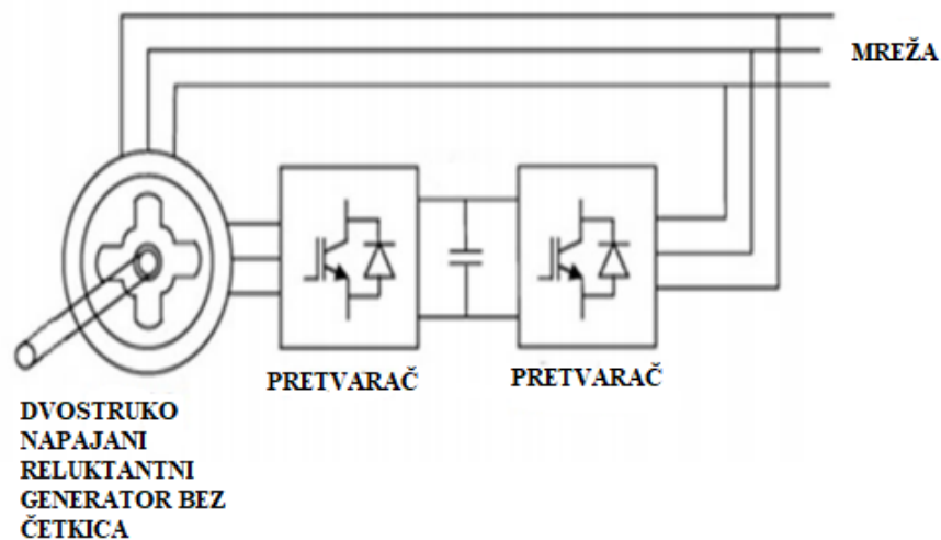
Slika 3.16. Shema spajanja dvostruko napajanih reluktantnih generatora bez četkica na mrežu [13]
